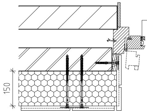
TOX wakkelplug
