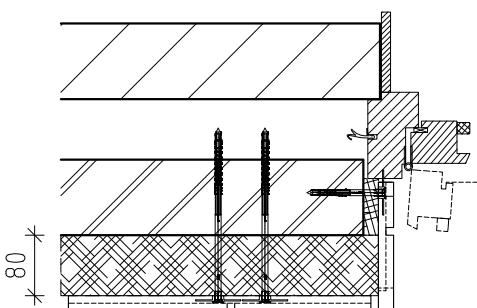
TOX wakkelplug
