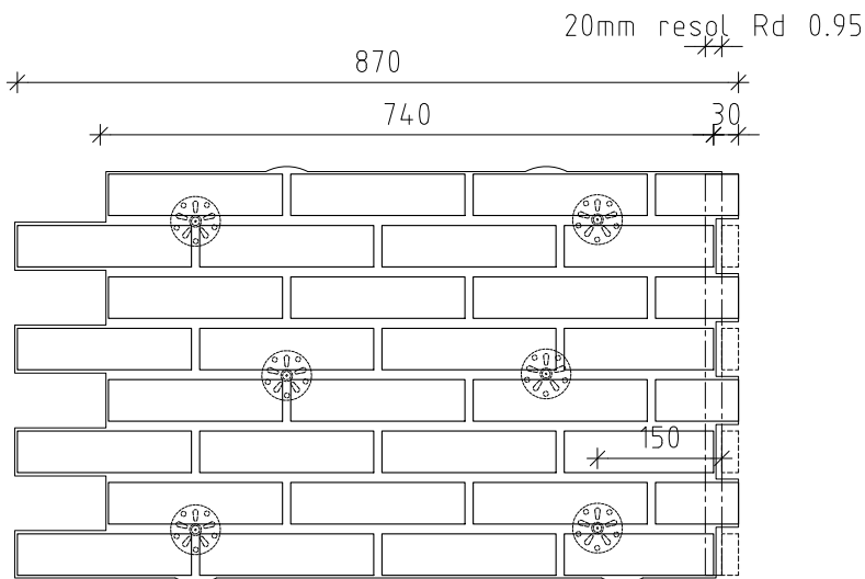
WF-HaV-xx-hoekpaneel 12 mm lintvoeg
