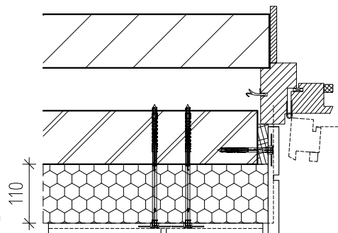
TOX wakkelplug
